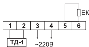
Схема подключения MPT220.12-16*
