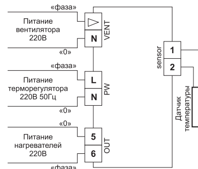
Схема подключения MPT220.14-16*
