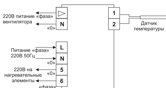
Схема подключения MPT220.10-16*
